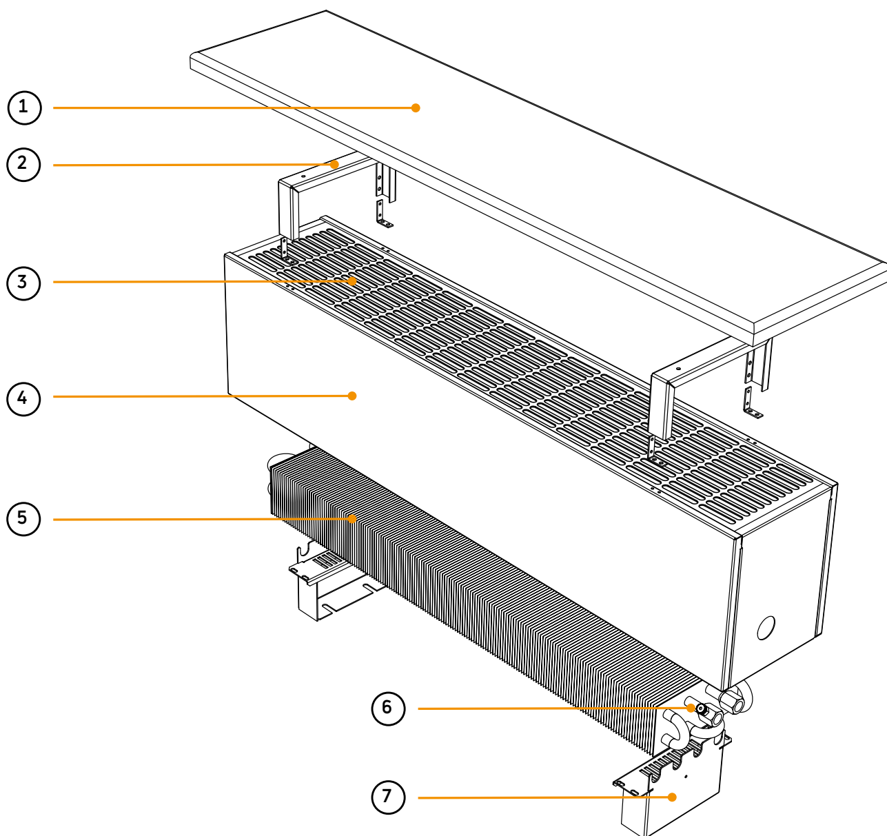
Konstrukcja grzejników Aura Bench WDF
