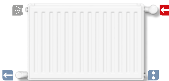
podłączenie krzyżowe
