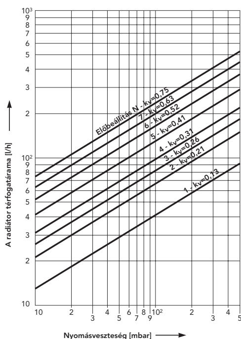
1. diagram: Nyomásvesztés [mbar] - kétsőves rendszerben 2K arányos eltérésnél
