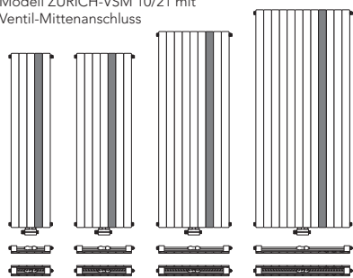
Modell ZÜRICH-VSM 10/21 mit Ventil-Mittenanschluss
