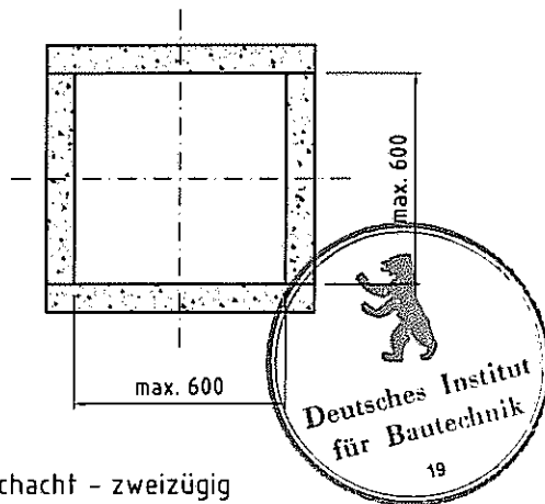
Schacht - einzügig
