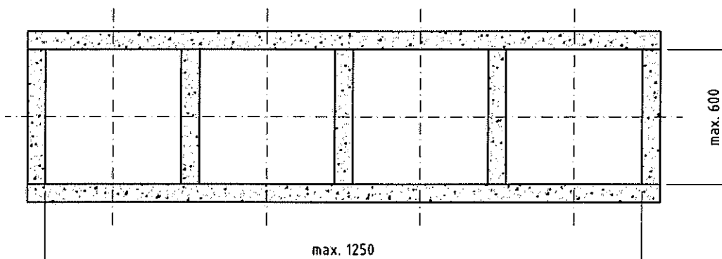
Schacht - mehrzügig
