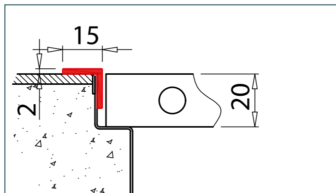
PML – L-Rahmen Buche 1
