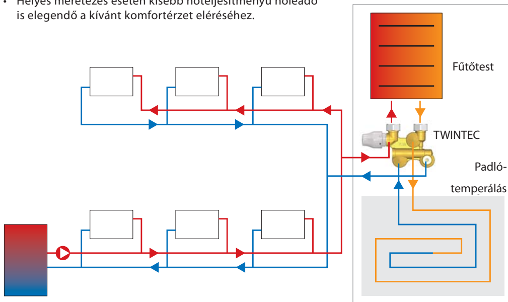
TWINTEC - lapradiátorhoz csatlakoztatva
