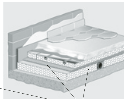
Zusatzdämmungen
