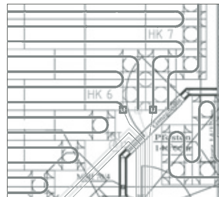
Erker-/Schrägausführung
