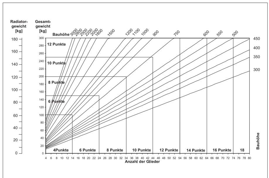
Abb. 3 Ermittlung der notwendigen Befestigungspunkte für 5- und 6-Säuler. Je ein Befestigungspunkt oben (empfohlene Position direkt unter der Nabe) und ein Befestigungspunkt unten (Abb. 1) bilden eine vertikale Befestigungsachse.
