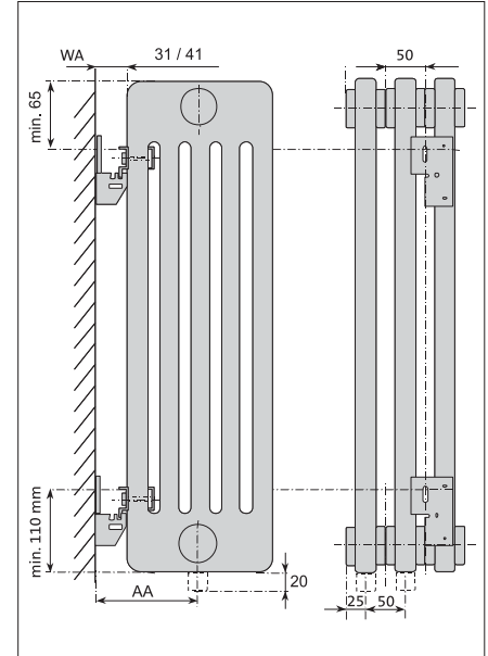
Abb. 1 Befestigung und Anschlußmaße für Anschluß-Set mit Winkelkonsole. Das 4er Set beinhaltet je viermal, das 6er Set je sechsmal den unten rechts abgebildeten Umfang
